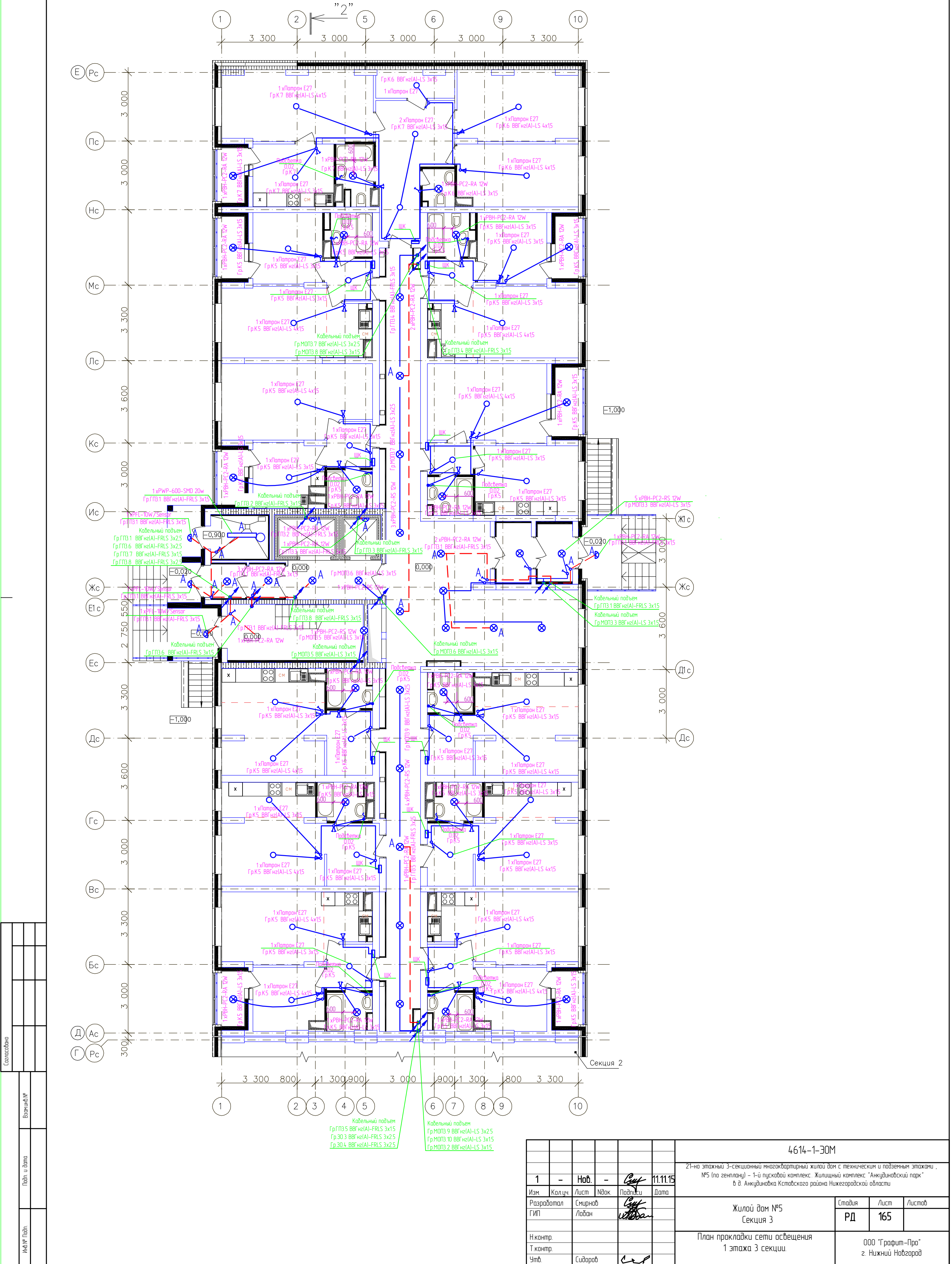
Отделочный план 1 этажа (отм.0,000) в осях 1–10/Д–Е. Секция 3
